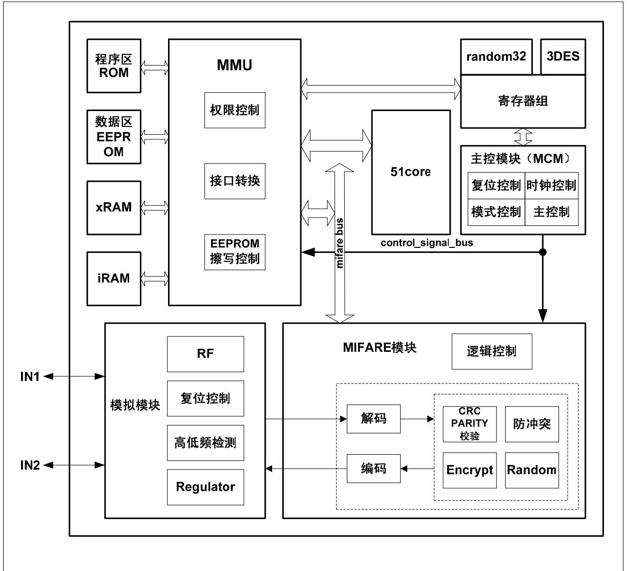
图 1-1 FM1208M01 功能框图
