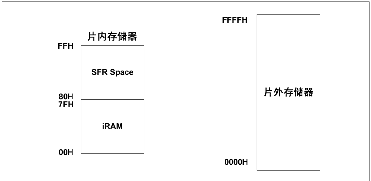
图 3-1 FM1208M01 存储器空间
