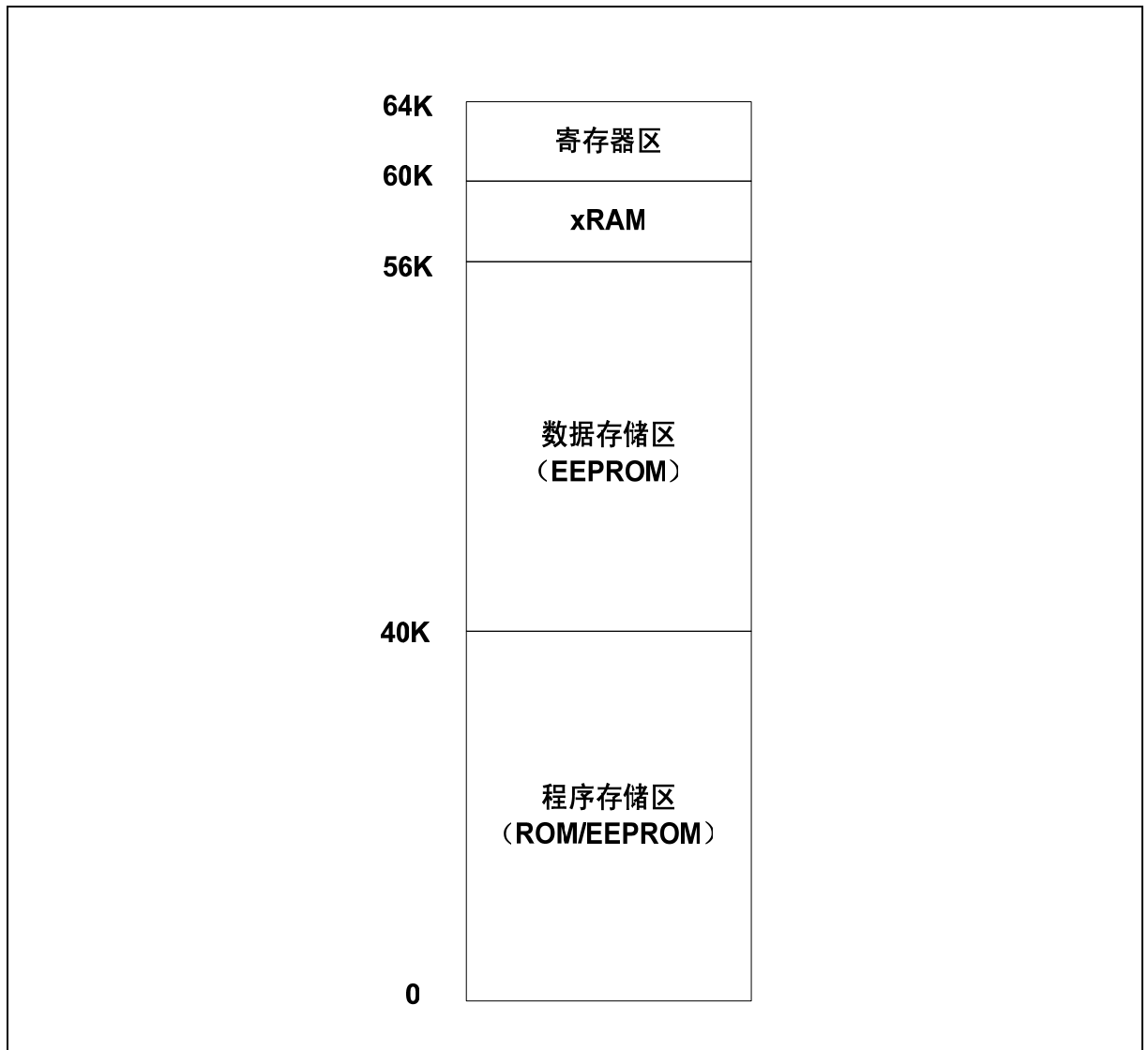
图 3-2 FM1208M01 片外存储器空间分配
