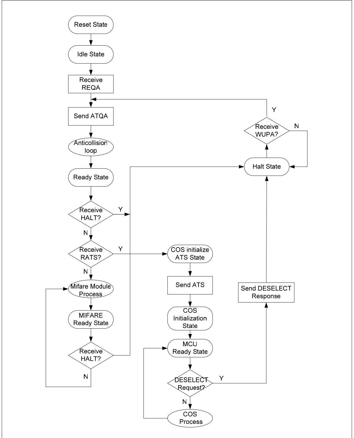
图 2-1 FM1208M01 芯片工作流程
